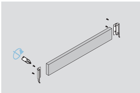
Montaż tylnej ścianki Back assembly
