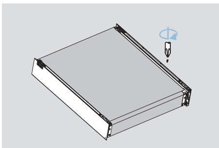
Przykręć śruby Fix screws
