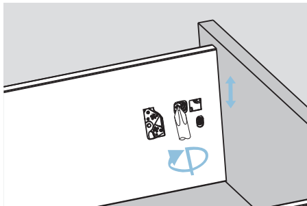
Regulacja pionowa Up&down adjustment
