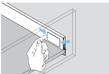
Zdejmij plastikowe zaślepki Remove cover caps
