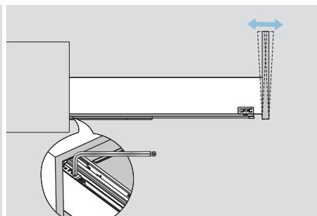
Regulacja nachelenia frontu (za pomocą klucza imbusowego M3) Tilt adjustment (by M3 Allen key)
