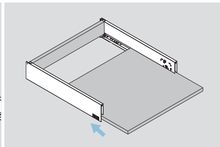
Montaż spodu szuflady Bottom assembly
