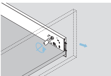
Użyj śrubokręta by zwolnić szufladę Turn screw driver to release the drawer front
